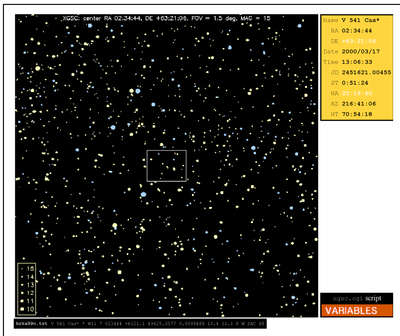
Obr. 3 — Ukázka z programu variables : vyhledávací mapa s hvězdami do 15. magnitudy (GSC katalog).
