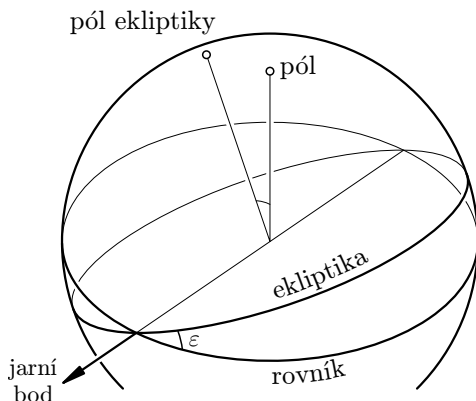
Obr. 4 — Soustavy rovníková II. druhu a ekliptikální.
