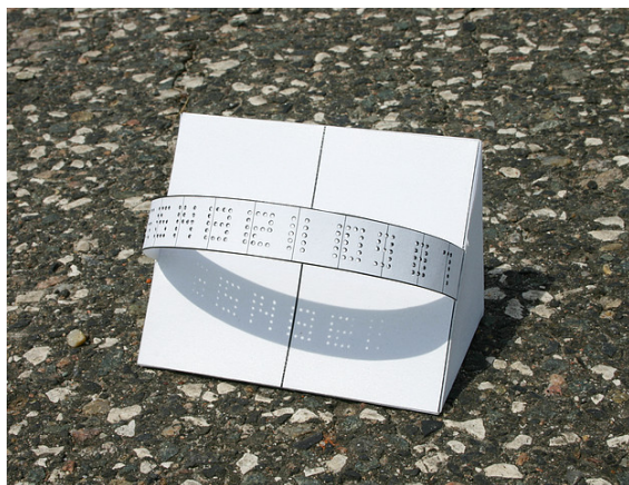
Obr. 8 — Splená vystřihovánka digitálních slunečních hodin.
