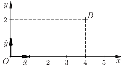
Obr. 1 — Bázové vektory a souřadnice v rovině.
