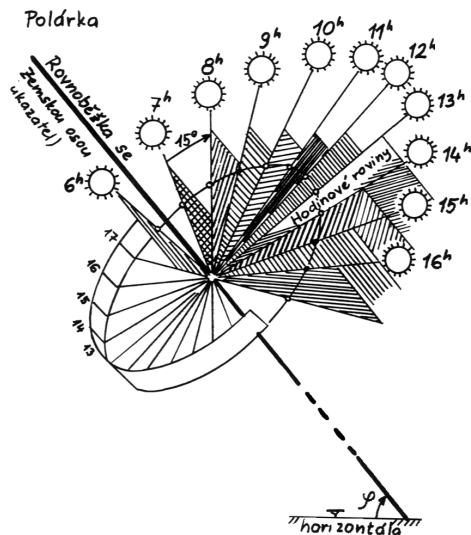
Obr. 9 — Denní pohyb Slunce po obloze a příslušné hodinové roviny.
