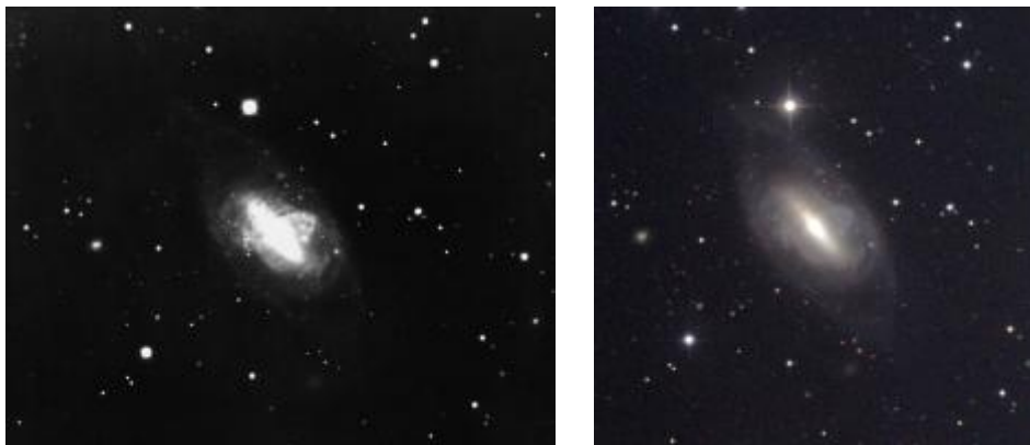
Obr. 5 — NGC 2685 na snímku z Kitt Peak National Observatory: (a) z roku 1975, Mayallovým dalekohledem o průměru 4 m; (b) 0,9 m dalekohledem z listopadu 1998. Převzato z [7], © AURA/NOAO/NSF, N.A. Sharp.
