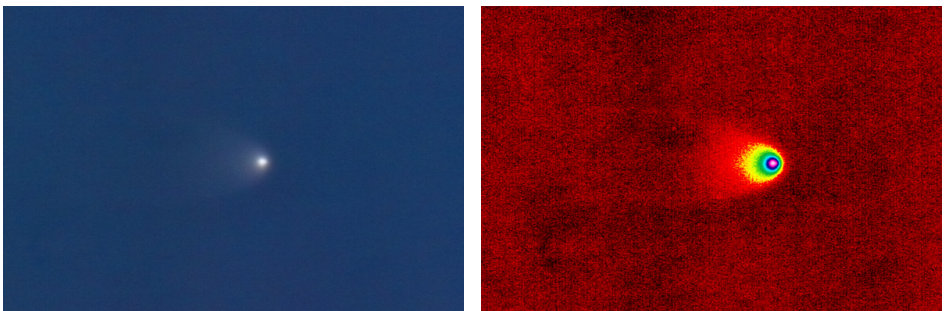
Obr. 19 — Kometa McNaught 14. 1. 2007 ve 12 h 30 min UT, Newtonem 210/1000 a aparátem Canon EOS 20D, s expozičními časy 5 krát 1/8000 s. Druhý snímek má převedené odstíny do barevné škály, pro zvýraznění rozložení jasu komety. Foto Martin Myslivec.
