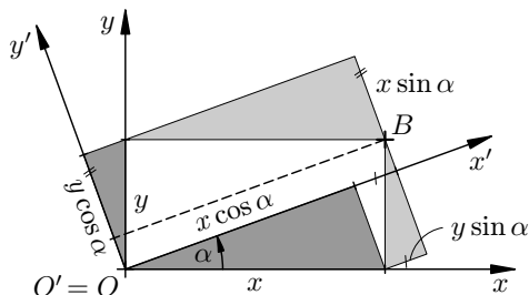
Obr. 2 — Otočení souřadnicové soustavy okolo počátku.
