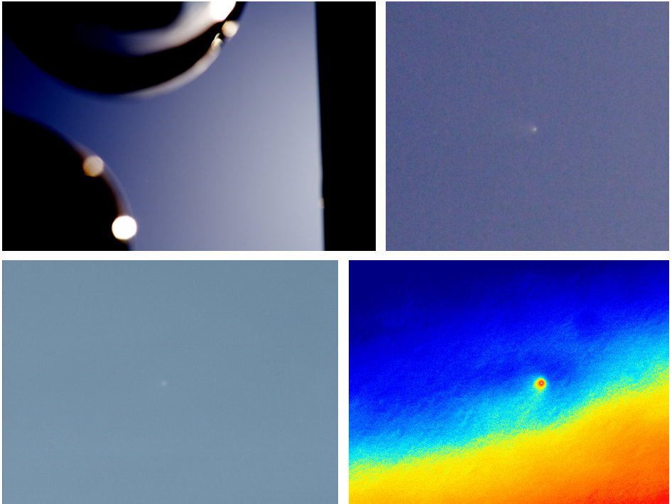
Obr. 18 — Několik snímků denní komety C/2006 P1 (McNaught) pořízených 14. 1. 2007 v 11 h 52 min UT (nahore), 15. 1. v 9 h 40 min a 14 h 9 min (dole) přístroji Canon Eos 300/350D s teleobjektivem Sigma DC 18–200 ( f = 200 mm) a v primárním ohnisku 20 cm refraktoru ( f = 3500 mm); po digitálním zpracování (programy Canon DPP, Iris, Photoshop CS, Gimp, Matlab). Foto Miroslav Brož.
