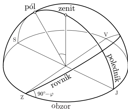
Obr. 3 — „Polokulový“ obrázek souřadnicových soustav obzorníkové a rovníkové I. druhu.
