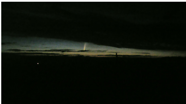
Obr. 15 — Kometa McNaught viděná 18. 1. 2007 v 10 h 49 min UT z Nového Zélandu; odhadovaná jasnost byla -4 mag. Přístroj Olympus C360Z, expoziční doba 2 s, f/3,1 , 400 ASA. Foto Miloslav Zejda.
