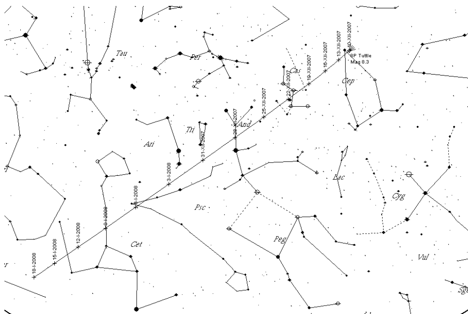
Obr. 10 — Dráha komety 8P/Tuttle na obloze v období od 10. prosince 2007 do 18. ledna 2008, kdy bude kometa nejlépe pozorovatelná. Polohy komety jsou vyneseny vždy pro 22:30 SEČ Na mapce jsou patrná výrazná souhvězdí podzimní a zimní oblohy (Peg – Pegasus, And – Andromeda, Cep – Kefeus, Per – Perseus, Cet – Velryba, Ari – Beran, Tau – Býk).
