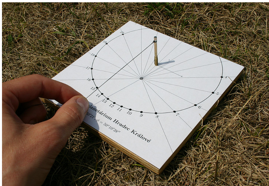
Obr. 6 — Sestavené hodiny stínové roviny.
