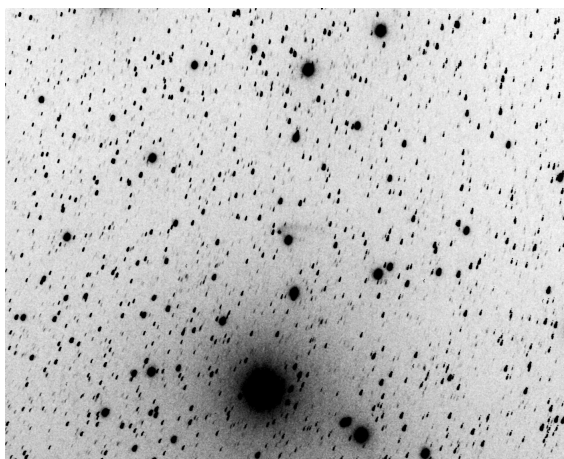
Obr. 4 — Planetka (596) Scheila snímaná 29. prosince 2010 v 7 h 25 min UT pomocí astrografu Takahashi FSQ 106, f/5 a CCD STL11K v Novém Mexiku. Jedná se o kompozici 5 \times 120 s. © Joseph Brimacombe.
