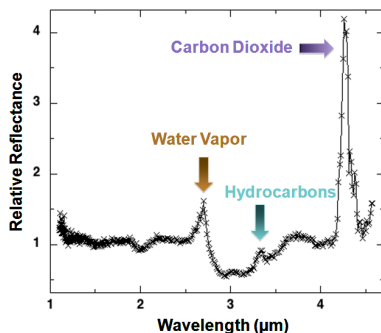
Obr. 2 — Infračervené spektrum získané přístrojem HRI. Označené jsou emise vody, uhlovodíků a oxidu uhličitého. © NASA/JPL-Caltech/UMD/McREL.
