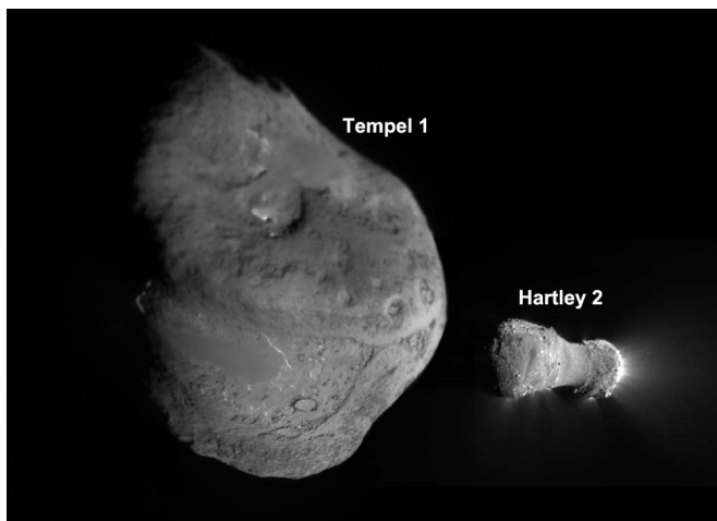
Obr. 1 — Porovnání kometárních jader 9P/Tempel 1 a 103P/Hartley 2 vyfotografovaných sondou Deep Impact/EPOXI. © NASA/JPL–Caltech/UMD/McREL.
