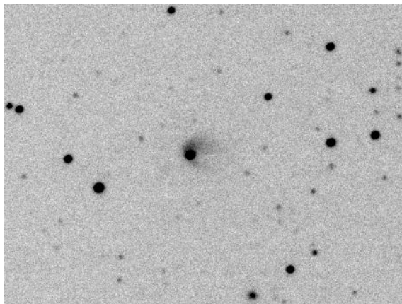
Obr. 3 — Snímek planetky (596) Scheila pořízený 12. prosince 2010 v 8 h 20 min UT pomocí reflektoru 0,25 m, f/3,4 a CCD kamety na observatoři GRAS (Mayhill, NM, USA). Jedná se o kompozici 8 \times 120 s. © Ernesto Guido a Giovanni Sostero.
