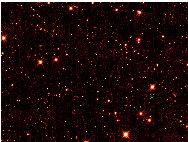
Obr. 2 — Snímek Trojana Země, pořízený v říjnu 2010 družicí WISE na vlnové délce 4,6 \mu\text{m} .
