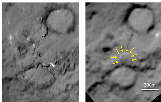
Obr. 4 — Impaktní kráter o průměru přibližně 150 m vytvořený penetrátorem vypuštěným ze sondy Deep Impact. © NASA, JPL–Caltech, University of Maryland, Cornell.
