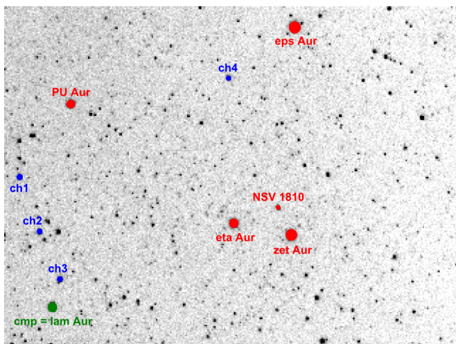
Obr. 7 — Snímek okolí \epsilon Aurigae pořízený CCD kamerou ST5–C přes objektiv Pentacon Auto 2,8/29 (zorné pole 379' \times 284' ). Vyznačené jsou proměnné hvězdy a srovnávací hvězdy (cmp, ch1 až ch4).
