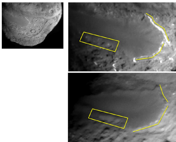
Obr. 3 — Porovnání snímků stejné části povrchu jádra komety 9P/Tempel 1 ilustrující působení sublimační eroze. Napravo nahoře je záběr z roku 2005 (Deep Impact) a pod ním z roku 2011 (Stardust NExT). © NASA, JPL–Caltech, University of Maryland, Cornell.
