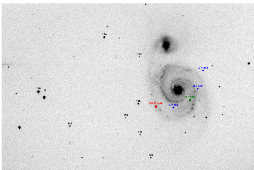
Obr. 5 — Snímek Vírové galaxie a supernovy 2011dh, pořízený 27. 6. 2011 pomocí dalekohledu JST (0,40 m, f/5 ) a CCD G2–1600 s filtrem R a expozicí 60 s (zorné pole je 24' \times 16' ). Vyznačené jsou srovnávací hvězdy podle AAVSO a kalibrované standardy podle práce Richmonda (1996).
