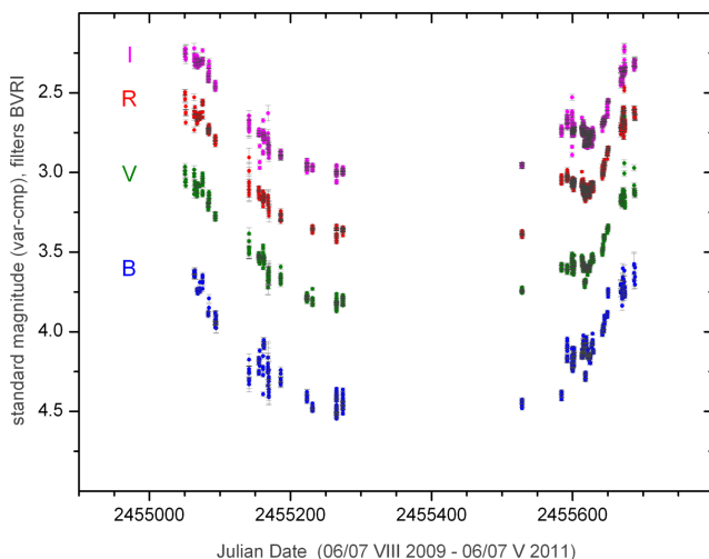
Obr. 8 — Světelná křivka \varepsilon Aurigae sestavená z měření pořízených během 60 nocí od 7. srpna 2009 do 6. května 2011.
