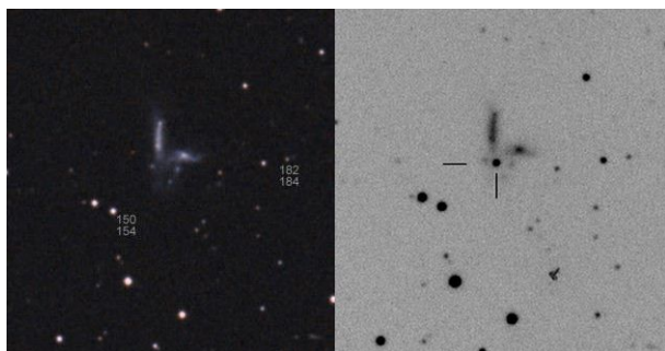
Obr. 9 — Vlevo snímek hostitelské galaxie UGC 3906 bez supernovy. Vpravo již se supernovou SN 2011aa v době objevu 6. 2. 2011. © Tim Puckett.
