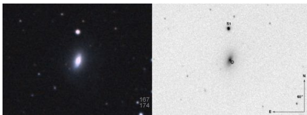
Obr. 17 — Vlevo snímek hostitelské galaxie UGC 2691 bez supernovy. Vpravo se supernovou SN 2011hr v době objevu 8. 11. 2011; převzato z ( http://astro.berkeley.edu/bait/public_html/2011/NGC2691.gif ).
