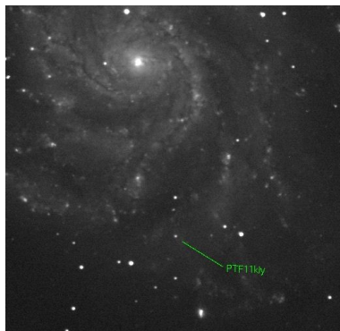
Obr. 15 — Snímek supernovy SN 2011fe v době objevu 24. 8. 2011. Převzato z ( http://www.cieletespace.fr/files/image_du_jour/snm101.jpg ).
