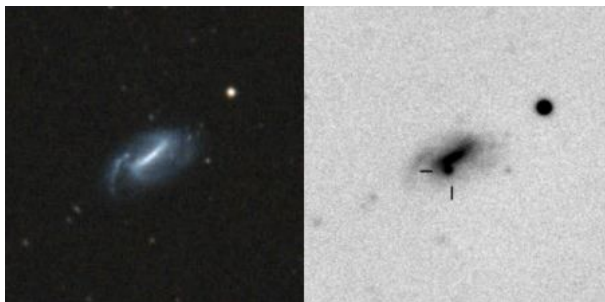
Obr. 11 — Vlevo snímek hostitelské galaxie IC 2973 bez supernovy. Vpravo je snímek se supernovou SN 2011ao v době objevu 3. 3. 2011. © Tim Puckett.
