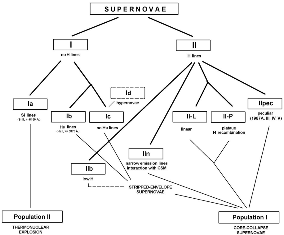
Obr. 18 — Klasifikační schéma supernov. Převzato z [2].
