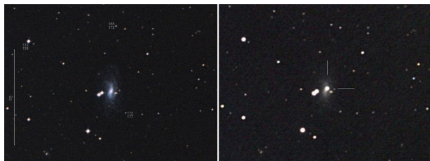
Obr. 10 — Vlevo snímek hostitelské galaxie MCG-03-30-19 zatím bez supernovy. Vpravo se supernovou SN 2011ae ze dne 9. 3. 2011. © Joseph Brimacombe; převzato z ( http://www.flickr.com/photos/43846774@N02/5513699511/ ).
