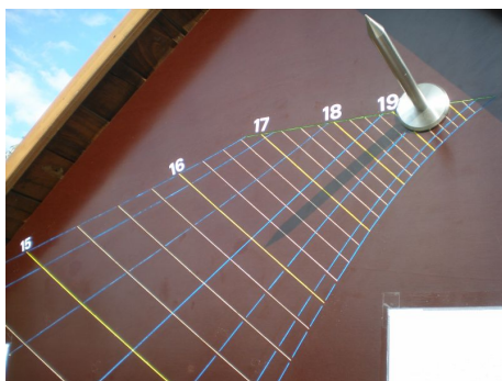
Obr. 19 — Západní sluneční hodiny ve Žlutavě (ZL 20). Foto V. Zíka.
