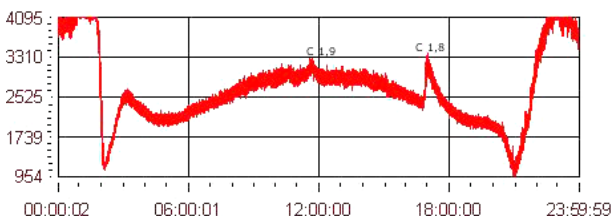
Obr. 4 — Záznam z hradecké observatoře zachycující dvě ionosférické poruchy – erupce.
