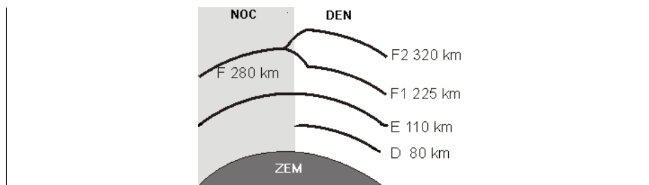
Obr. 1 — Schéma vrstev ionosféry Země.
