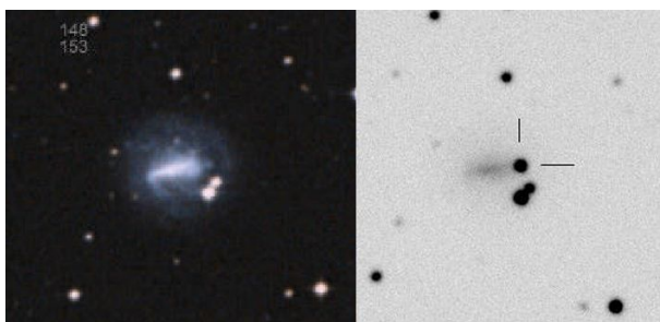
Obr. 12 — Vlevo snímek hostitelské galaxie MCG-02-24-27. Vpravo se supernovou SN 2011at v době objevu 10. 3. 2011. © Tim Puckett.
