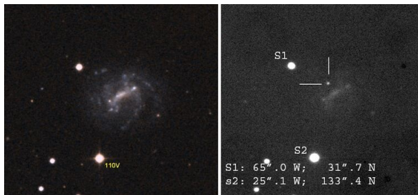
Obr. 16 — Vlevo snímek hostitelské galaxie UGC 5460 bez supernovy. Vpravo se supernovou SN 2011ht, tehdy ještě známou pouze pod názvem PSN J10081059+5150570, v době objevu 29. 9. 2011. © Tom Boles.
